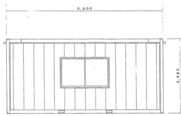
Y2立面図 S=1/50
